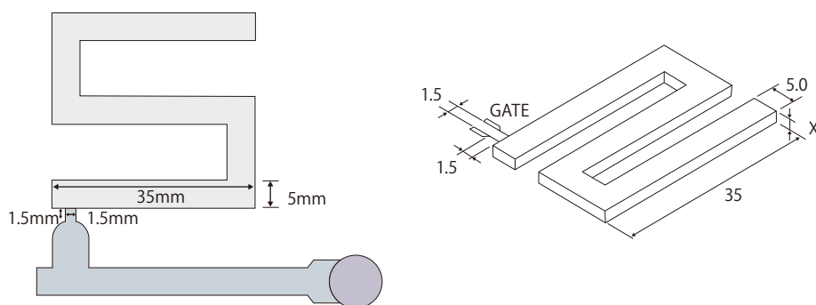
図 4-2-7 薄肉流動長
