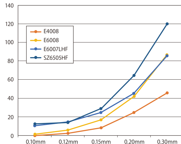
図 4-2-9 薄肉流動長の厚み依存性2
