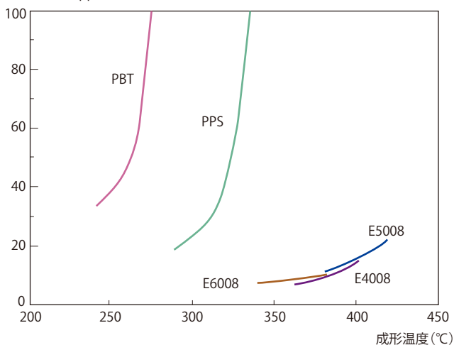
図 3-5-2 スミカスーパー LCP の発生ガス量
