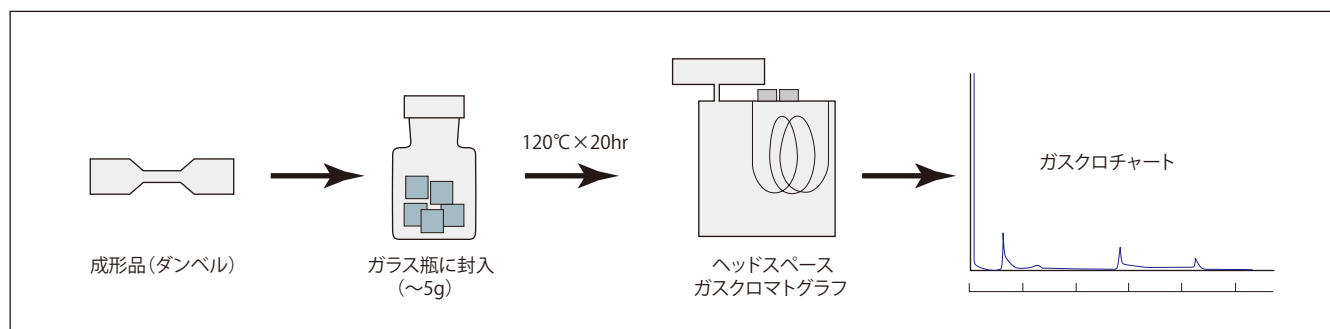
図 3-5-2 スミカスーパー LCP の発生ガス量
