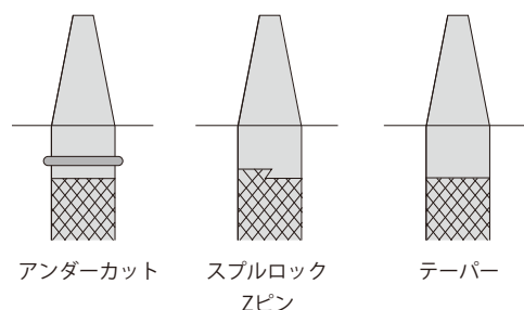
図 4-3-4 スプル図
