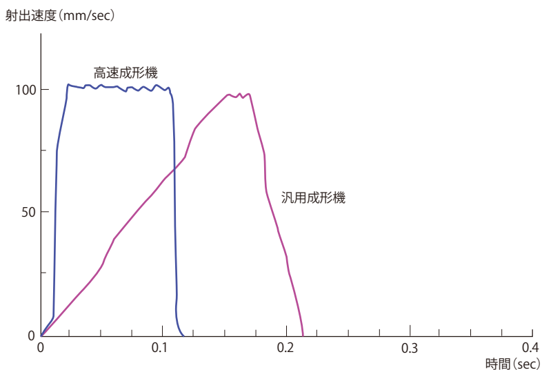
図 4-3-3 射出速度波形の比較
