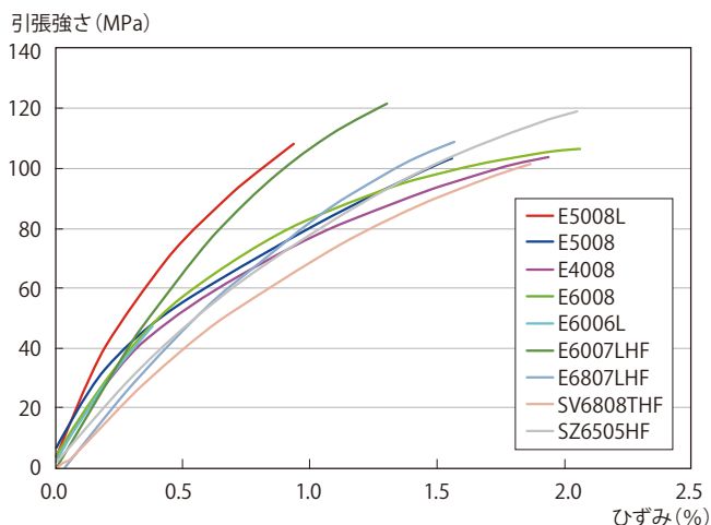
図 3-2-1 スミカスーパー LCP の S-S カーブ (室温)
