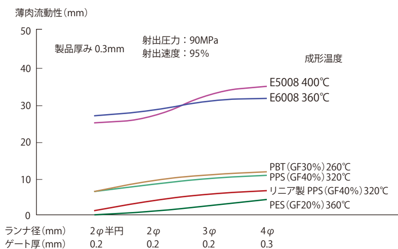
図 4-3-6 薄肉流動長
