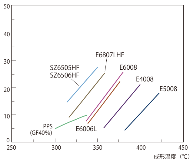
図 4-2-5 各種エンプラの 1mm 厚みの流動性
