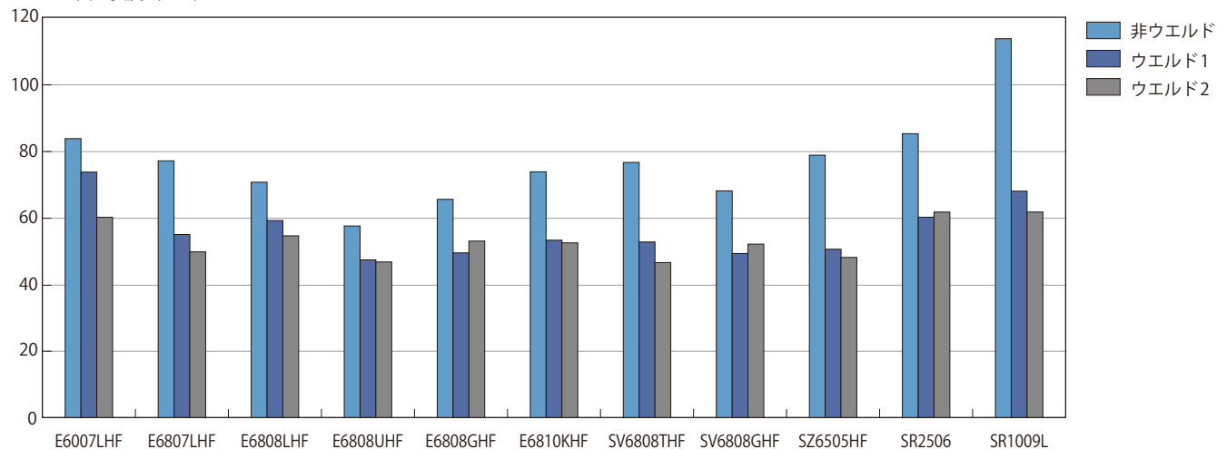
図 3-2-9 スミカスーパー LCP のウエルド曲げ強度 (0.5mm 厚み)
