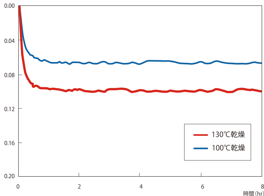
図 4-1-1 スミカスーパー LCP の乾燥曲線
