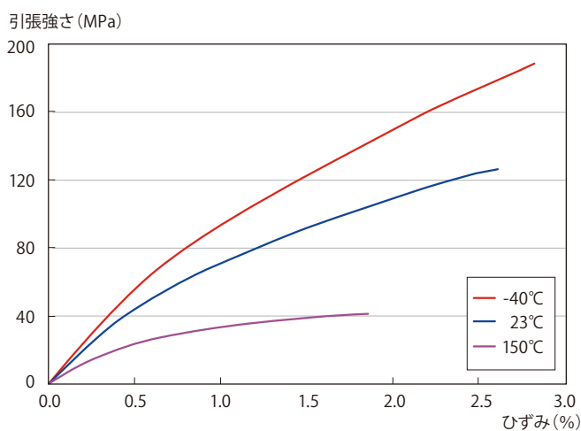
図 3-2-2 E6008 の引張強さの温度依存性
