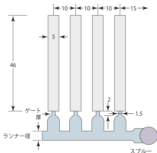
図 4-2-3 薄肉流動長測定金型 (単位: mm)
