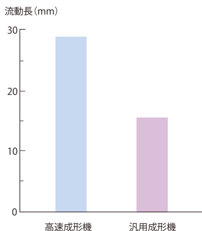
図 4-3-2 バリ発生を伴わない最大流動長
