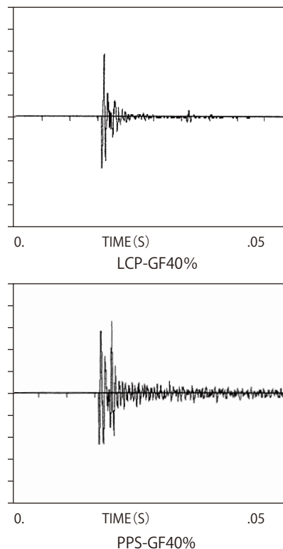
図 3-7-2 LCP と PPS の振動減衰性の比較
