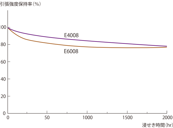
図 3-1-4 スミカスーパー LCP の耐熱水性 (80℃)
